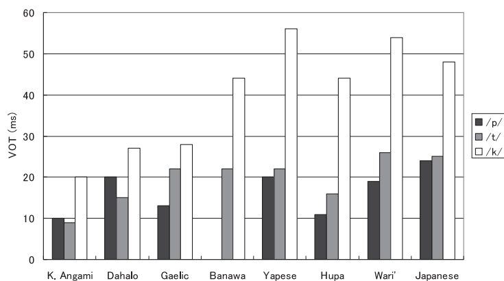
図2 8言語のVOT (Cho & Ladefoged, 1999のデータに基づく)
