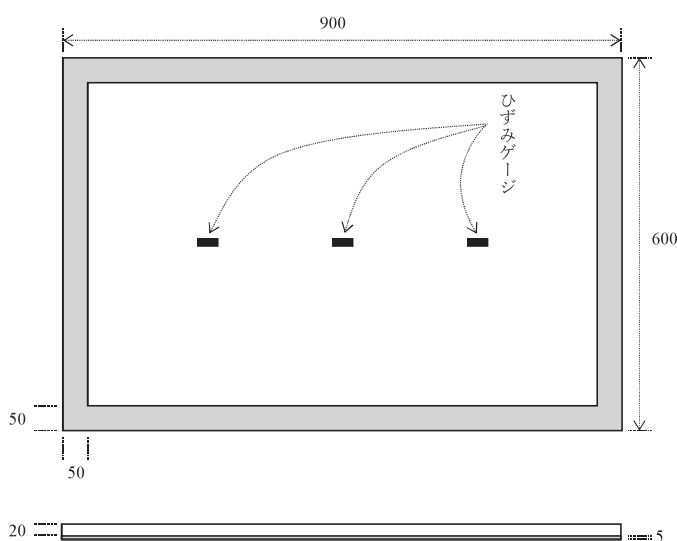
図1 アクリル板（900×600×20mm）にひずみゲージを貼付してジャンプ中の接地時間と跳躍時間を検出。 左から1ch, 2ch, 3chのひずみ信号を計測する。
